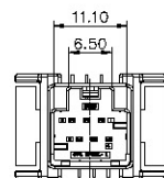
2*03PIN
